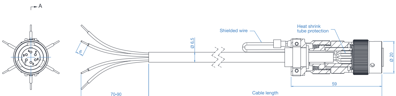
VIEW A-A
